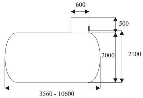
Samletanker type SL 10 m 3 til 32 m 3
