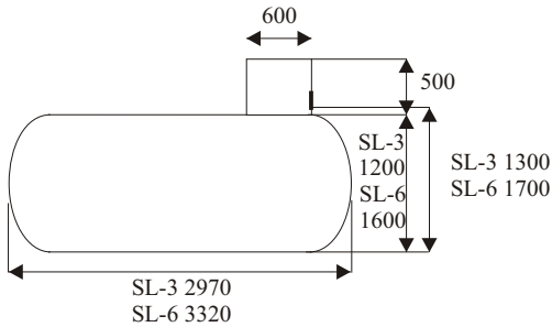
Samletanker type SL 3 m 3 og 6 m 3
