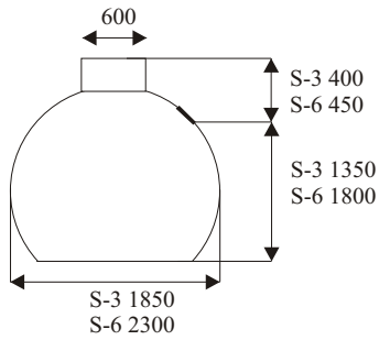
Samletanker type S 3 m 3 og 6 m 3
